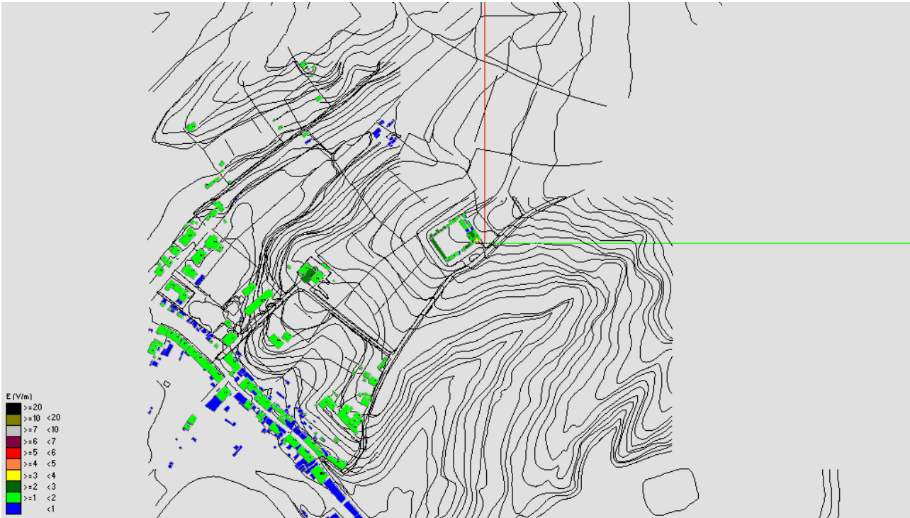
Fig. 57 Impatto elettromagnetico – Zona Cimitero Fontanella– Vista dall'alto
