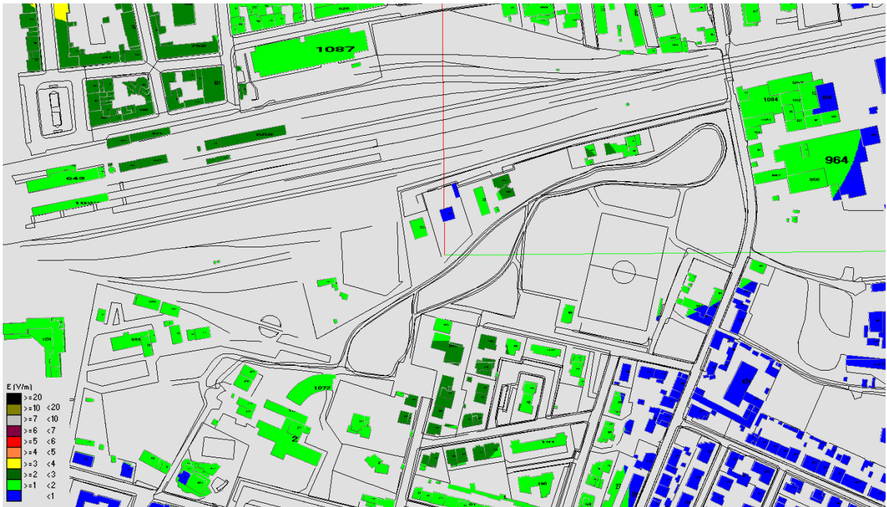
Fig. 33 Impatto elettromagnetico – Zona Via Nobile – Vista dall'alto
