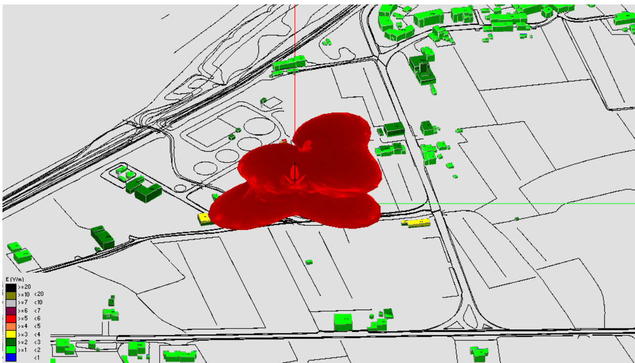
Fig. 14 Impatto elettromagnetico – Zona Cimitero Pagnana – 0°/Nord
