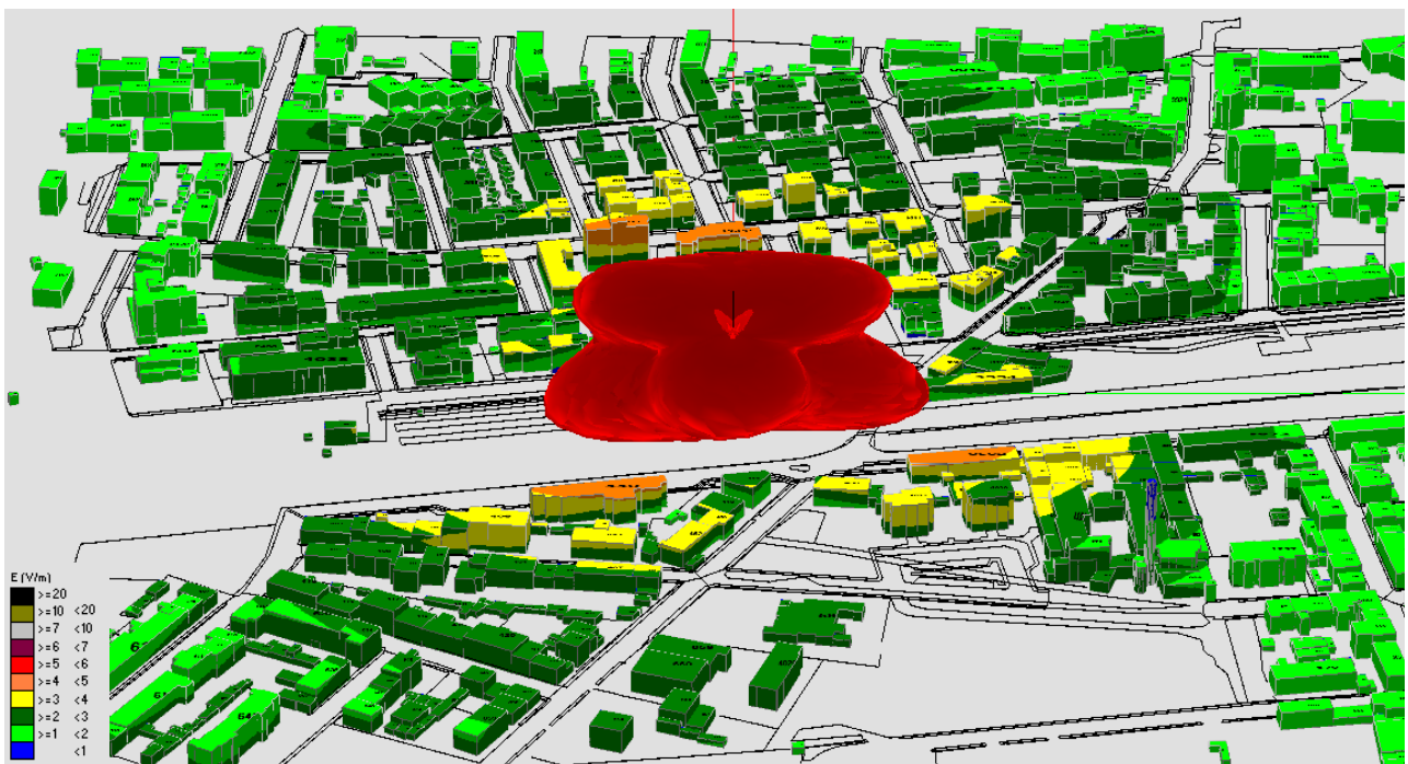
Fig. 29 Impatto elettromagnetico – Zona Via Buozzi – 0°/Nord
