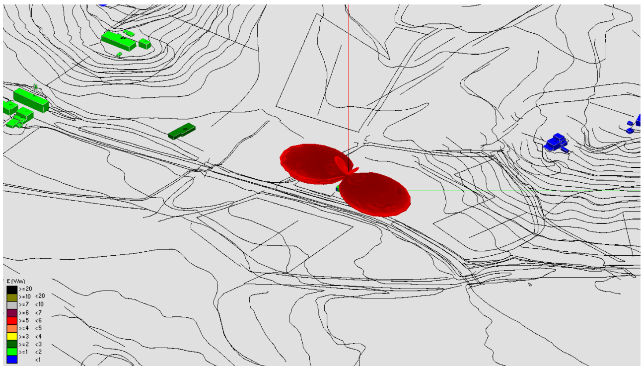
Fig. 53 Impatto elettromagnetico – Zona Cimitero Martignana – 0°/Nord
