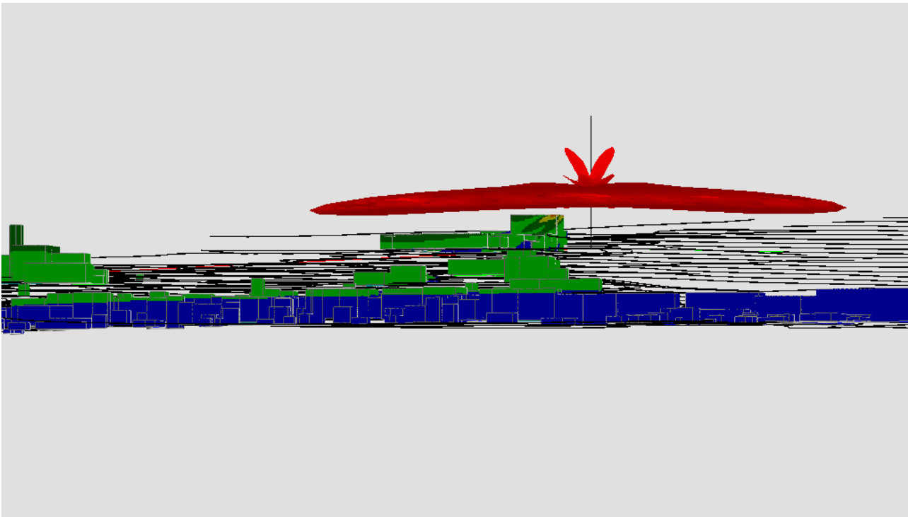
Fig. 58 Impatto elettromagnetico – Zona Cimitero Fontanella – Vista Laterale
