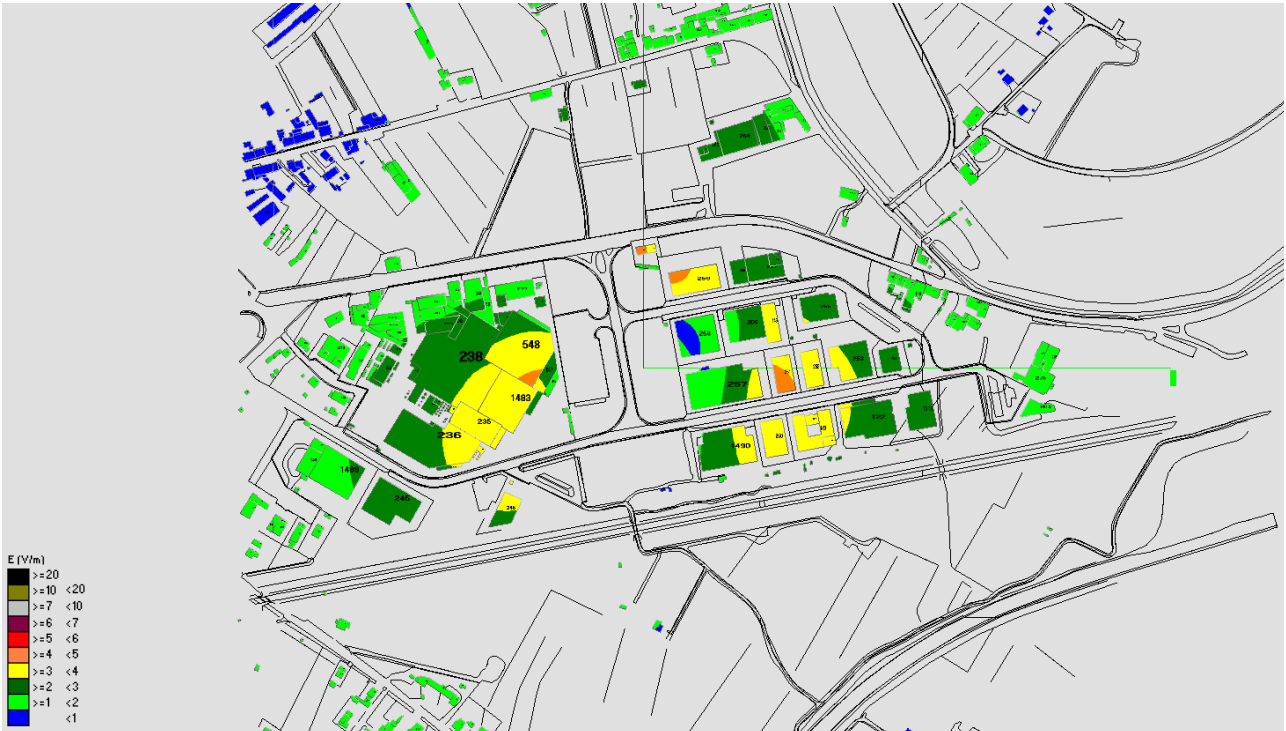
Fig. 21 Impatto elettromagnetico – Zona Pontorme – Vista dall'alto
