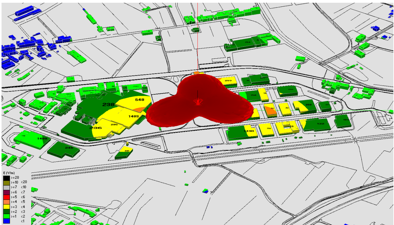
Fig. 20 Impatto elettromagnetico – Zona Pontorme – 0°/Nord
