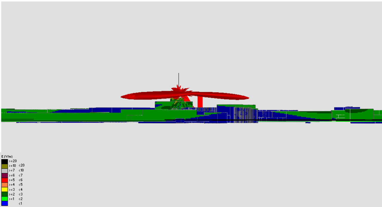
Fig. 40 Impatto elettromagnetico – Zona Terrafino - SS67 – Vista Laterale
