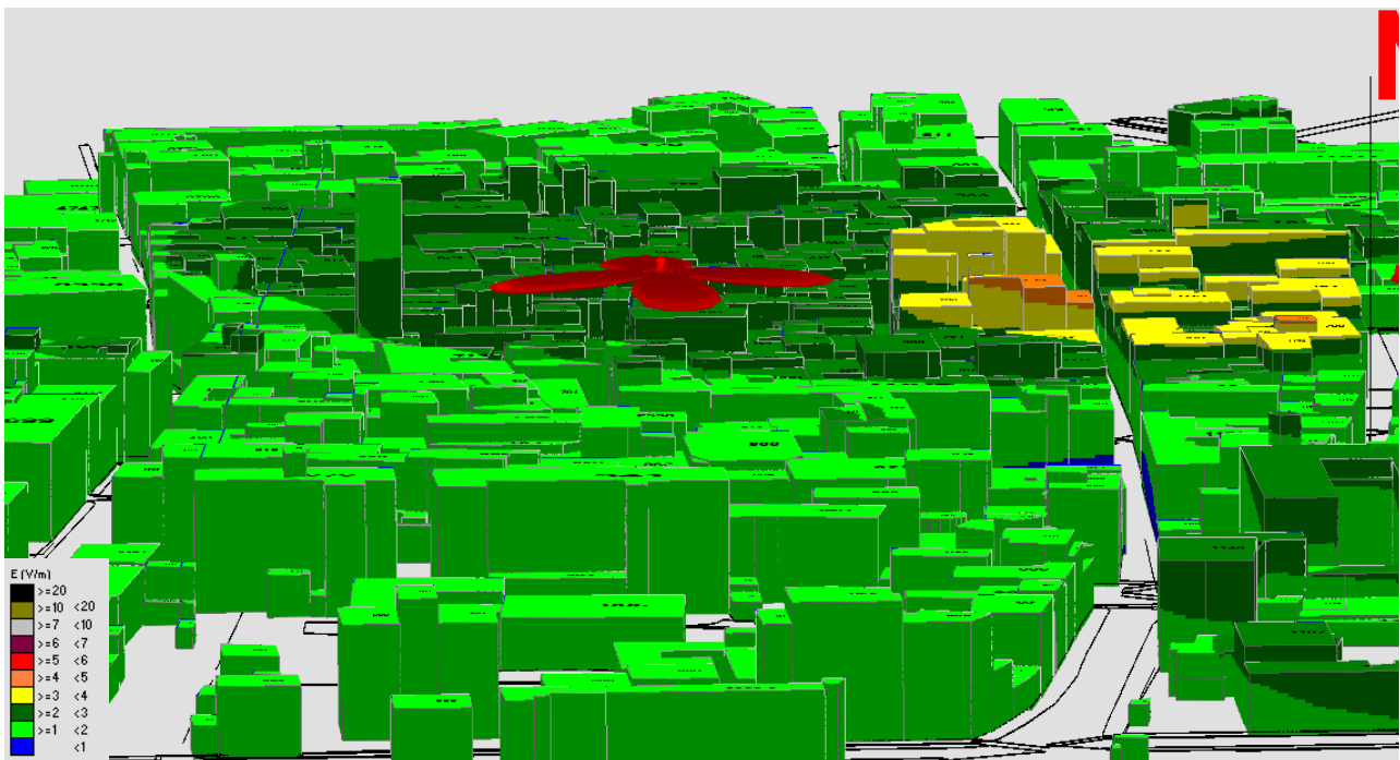
Fig. 12 Impatto elettromagnetico – Zona Empoli Centro H3G – Vista Laterale
