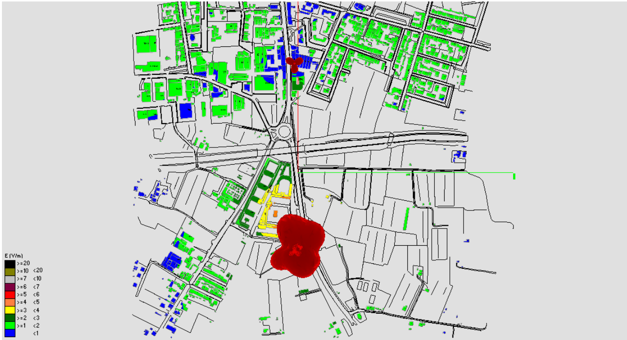
Fig. 44 Impatto elettromagnetico – Zona Via dei Cappuccini –Vista dall'alto
