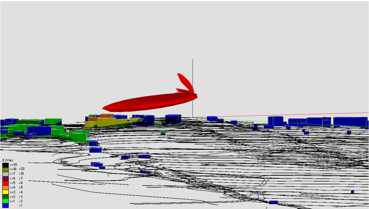
Fig. 52 Impatto elettromagnetico – Zona Monterappoli – Vista Laterale
