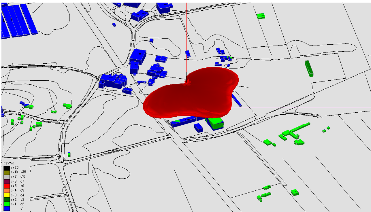
Fig. 47 Impatto elettromagnetico – Zona Cimitero Ponte a Elsa – 0°/Nord
