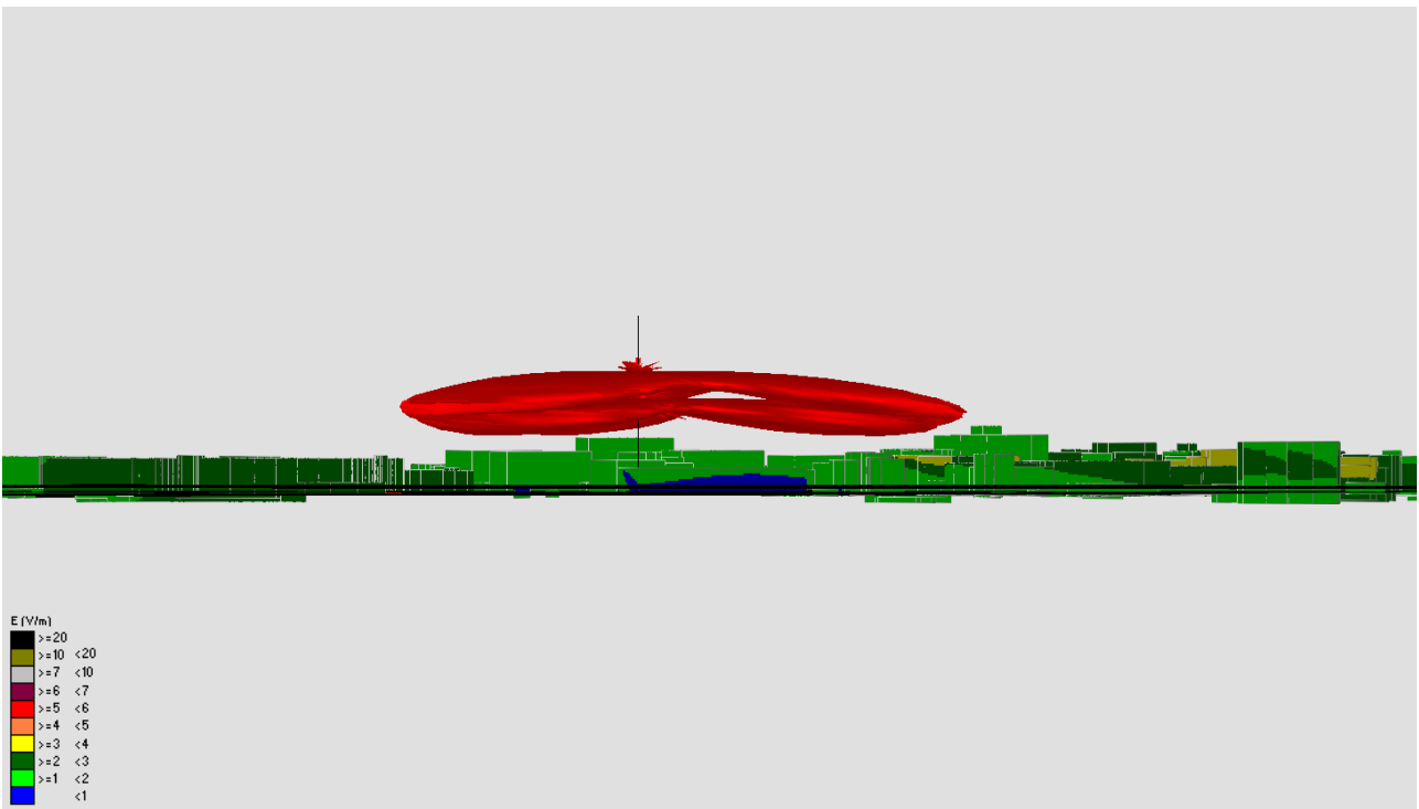
Fig. 28 Impatto elettromagnetico – Zona Via Majorana – Vista Laterale
