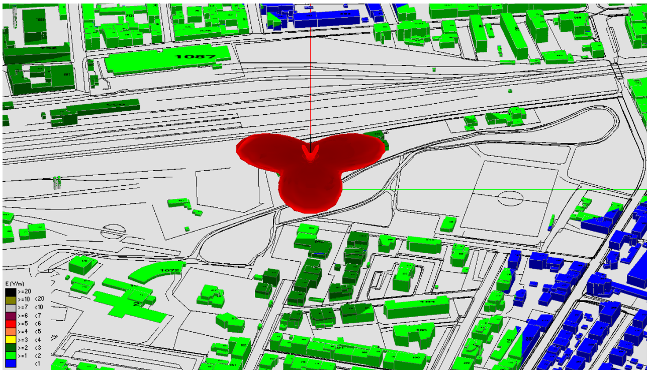
Fig. 32 Impatto elettromagnetico – Zona Via Nobile – 0°/Nord
