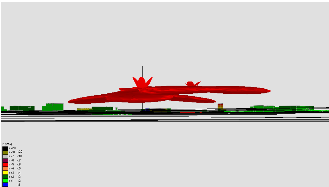
Fig. 16 Impatto elettromagnetico – Zona Cimitero Pagnana – Vista Laterale
