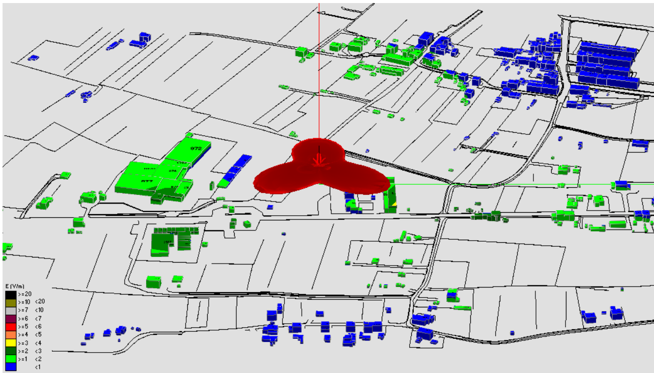
Fig. 17 Impatto elettromagnetico – Zona Cimitero S.Maria – 0°/Nord
