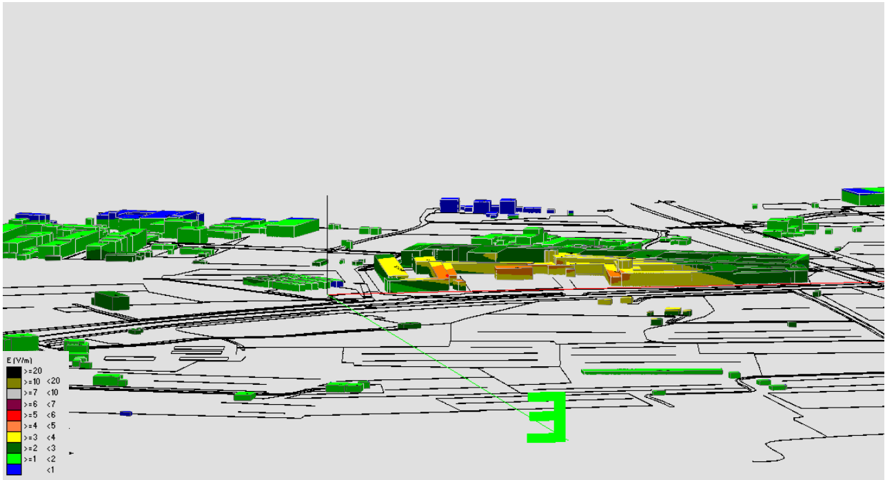
Fig. 46 Impatto elettromagnetico – Zona Cimitero Cappuccini TELECOM VODAFONE – Vista laterale
