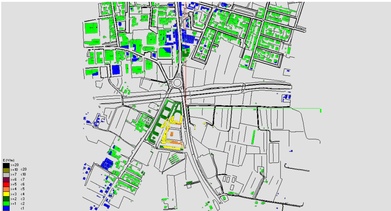
Fig. 45 Impatto elettromagnetico – Zona Via dei Cappuccini –Vista dall'alto
