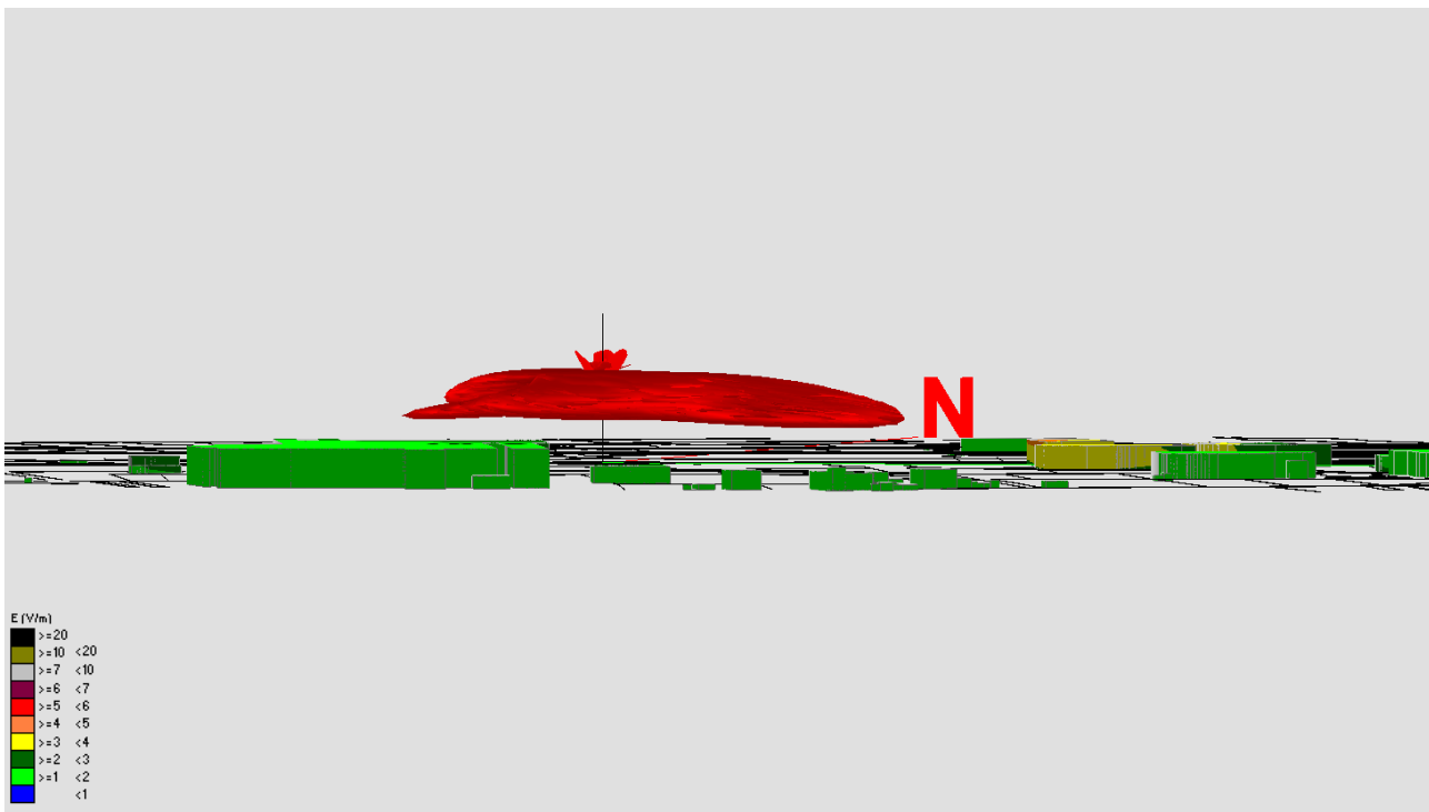
Fig. 37 Impatto elettromagnetico – Zona Terrafino Via I Maggio – Vista Laterale
