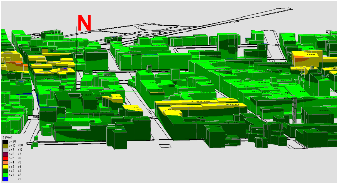
Fig. 13 Impatto elettromagnetico – Zona Empoli Centro TELECOM – Vista Laterale
