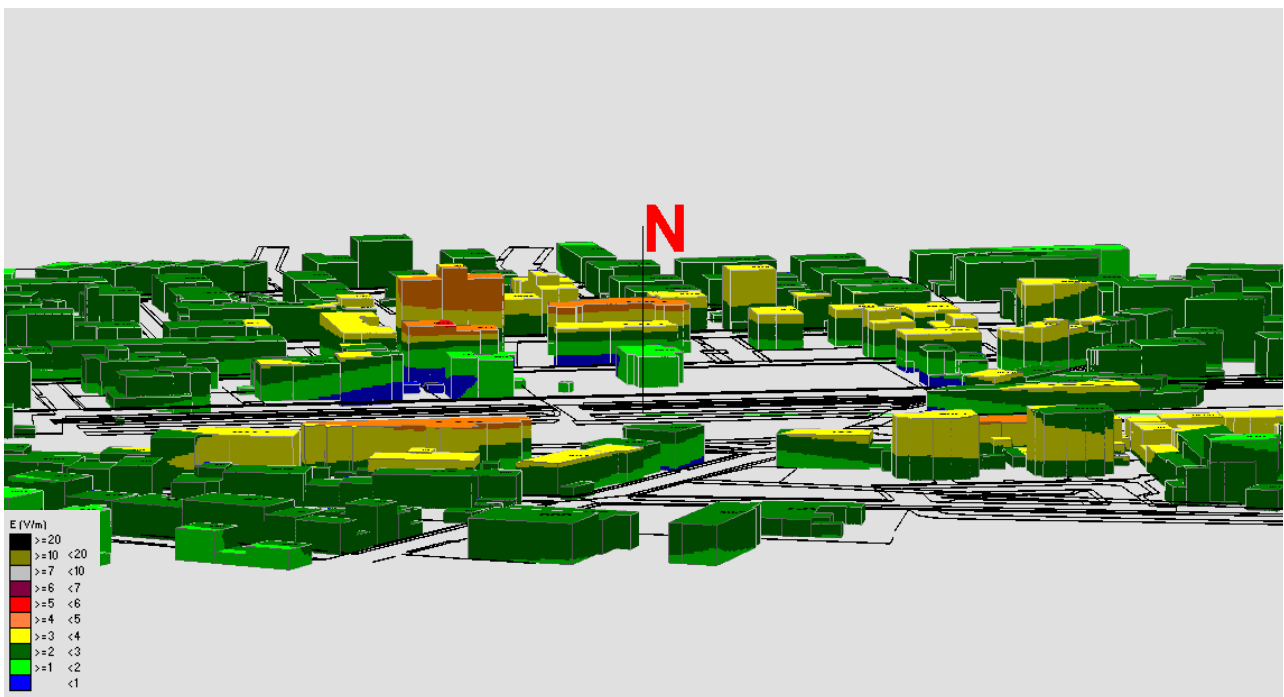
Fig. 31 Impatto elettromagnetico – Zona Via Buozzi – Vista Laterale
