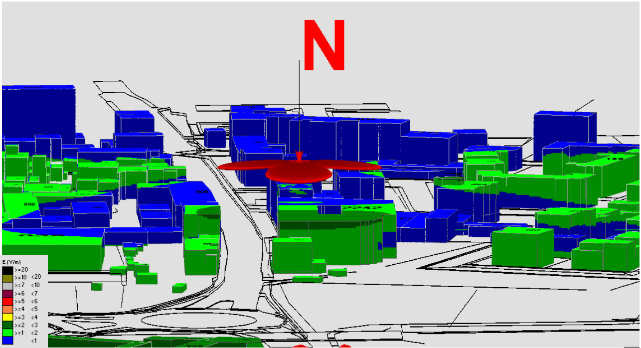
Fig. 42 Impatto elettromagnetico – Zona Via dei Cappuccini H3G –Vista laterale
