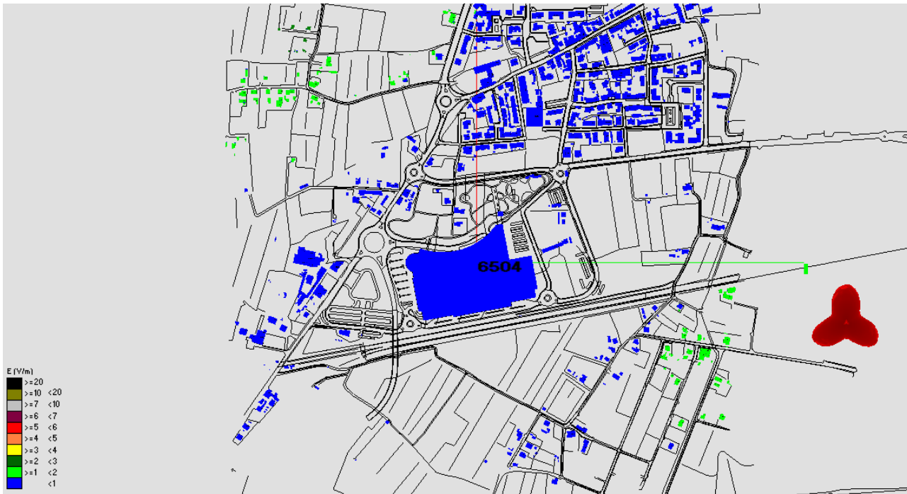
Fig. 24 Impatto elettromagnetico – Zona Centro Commerciale – Vista dall'alto
