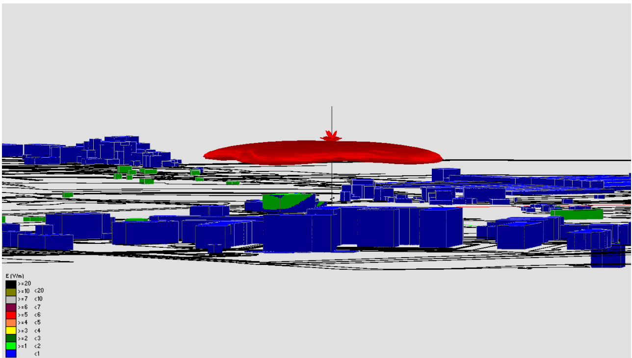
Fig. 49 Impatto elettromagnetico – Zona Cimitero Ponte a Elsa – Vista Laterale
