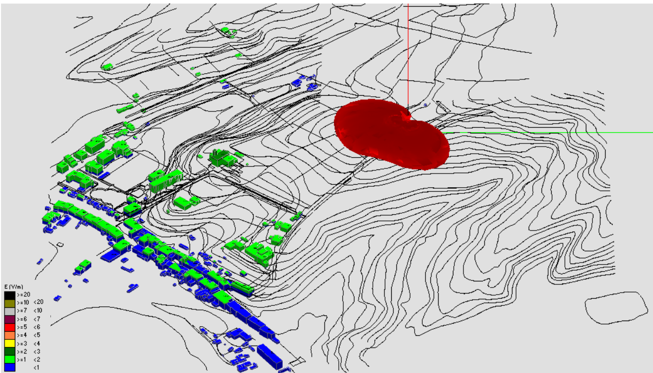
Fig. 56 Impatto elettromagnetico – Zona Cimitero Fontanella – 0°/Nord
