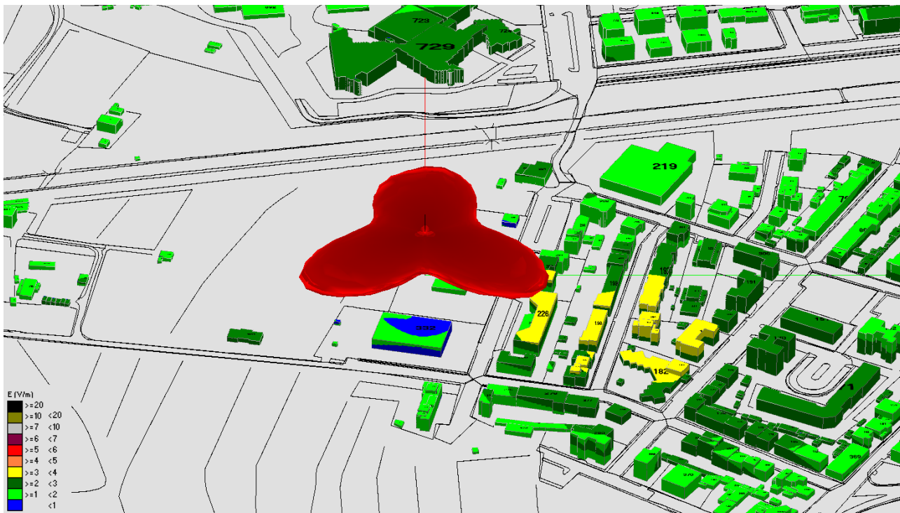
Fig. 26 Impatto elettromagnetico – Zona Via Majorana – 0°/Nord
