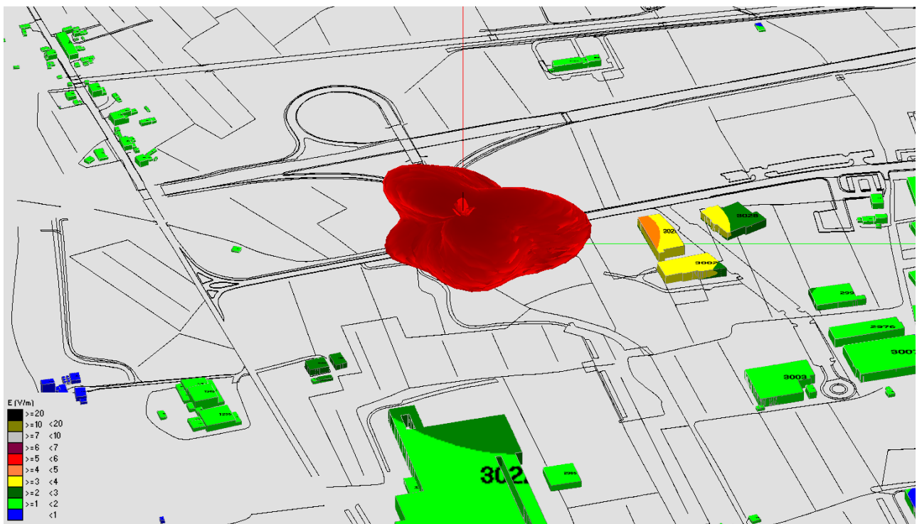
Fig. 35 Impatto elettromagnetico – Zona Terrafino Via I Maggio – 0°/Nord
