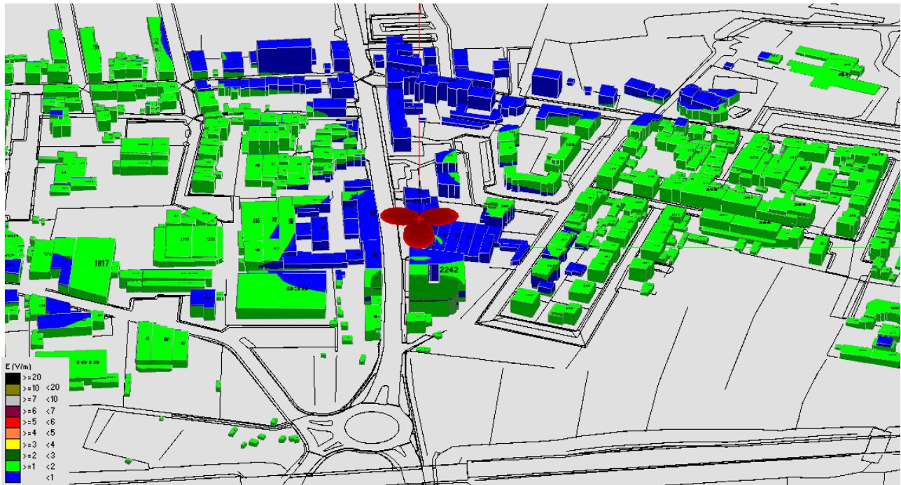
Fig. 41 Impatto elettromagnetico – Zona Via dei Cappuccini H3G – 0°/Nord
