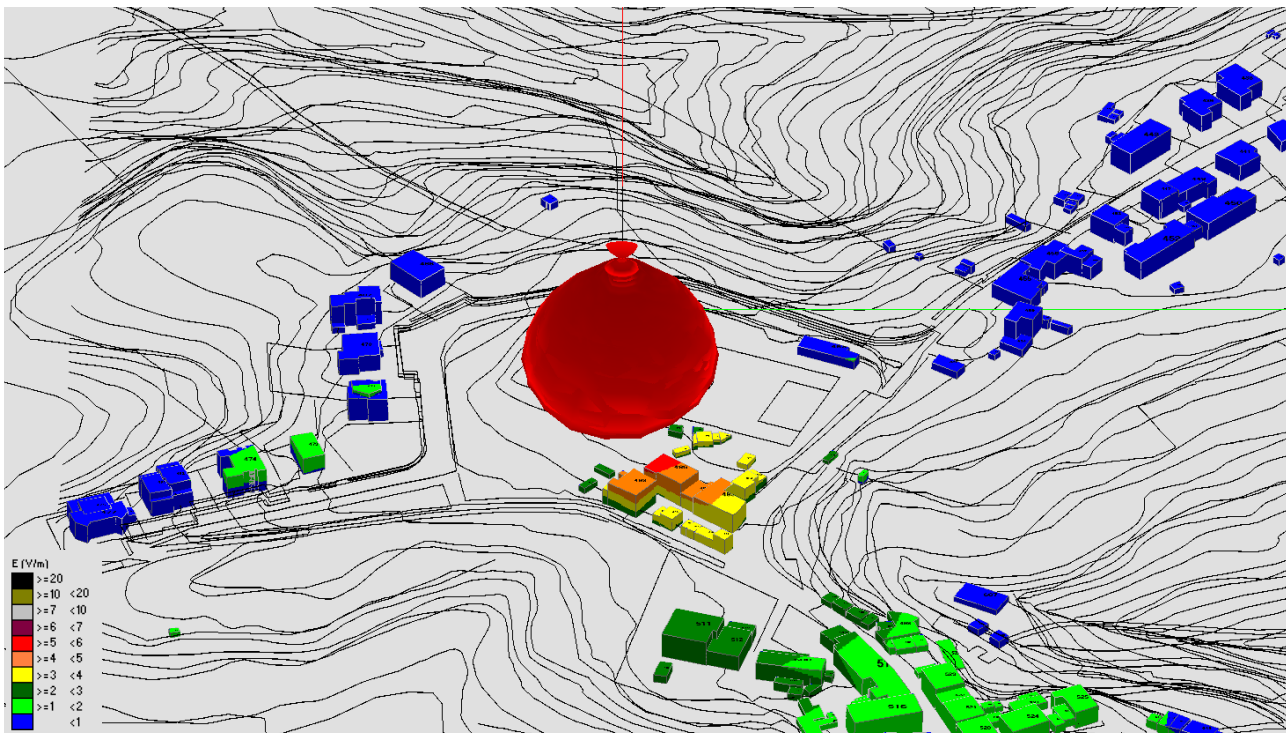
Fig. 50 Impatto elettromagnetico – Zona Monterappoli – 0°/Nord
