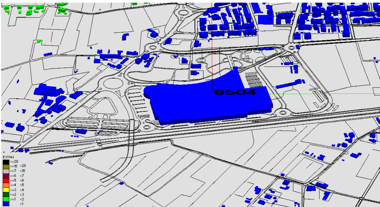
Fig. 23 Impatto elettromagnetico – Zona Centro Commerciale – 0°/Nord
