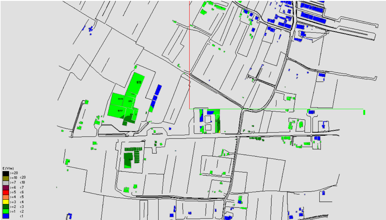
Fig. 18 Impatto elettromagnetico – Zona Cimitero S.Maria – Vista dall'alto
