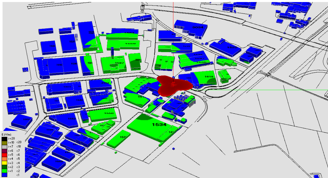
Fig. 38 Impatto elettromagnetico – Zona Terrafino - SS67 – 0°/Nord
