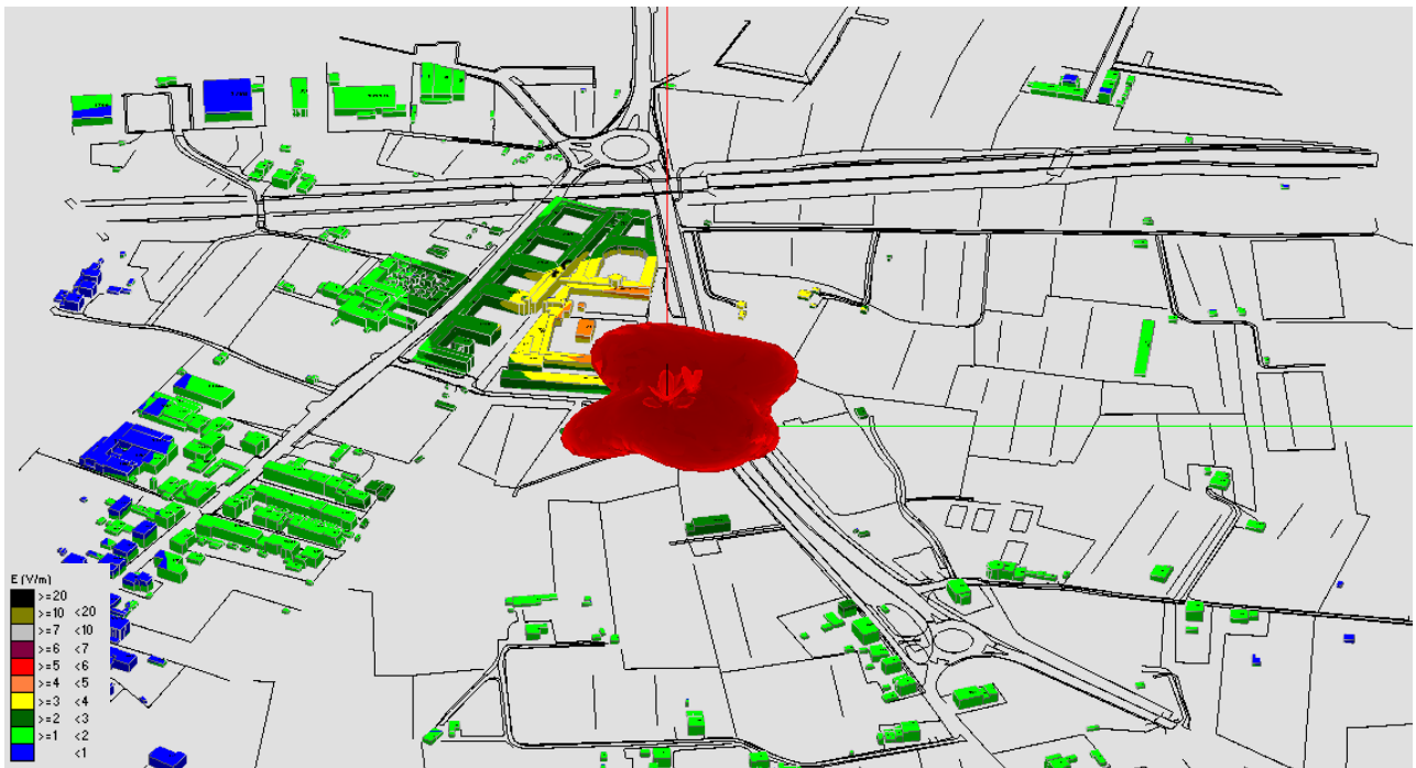
Fig. 43 Impatto elettromagnetico – Zona Via dei Cappuccini TELECOM – VODAFONE – 0°/Nord
