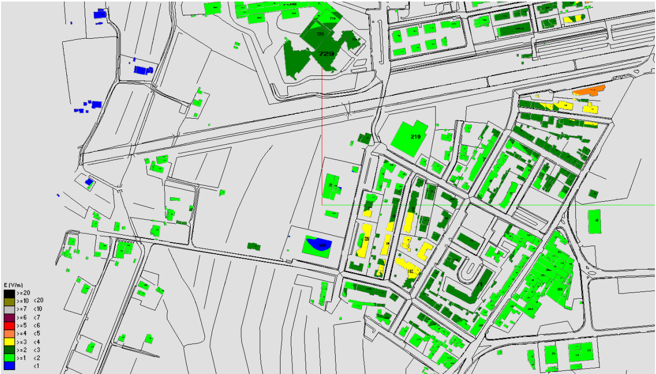
Fig. 27 Impatto elettromagnetico – Zona Via Majorana – Vista dall'alto
