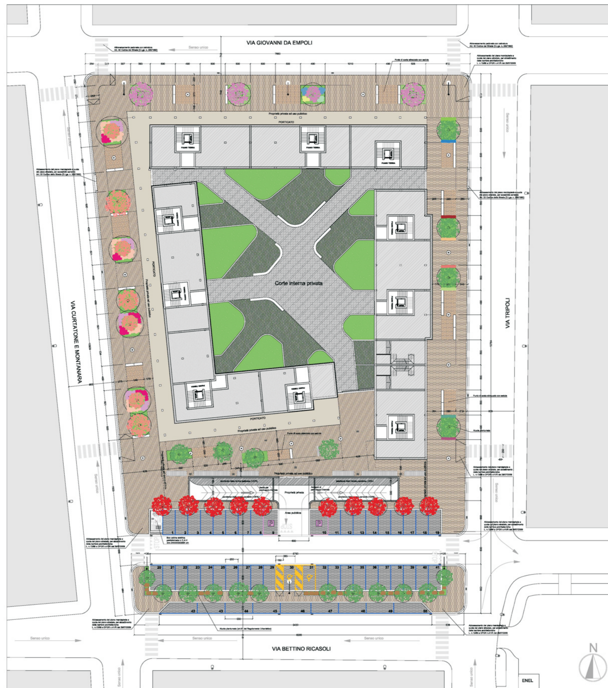
PLANIMETRIA GENERALE
