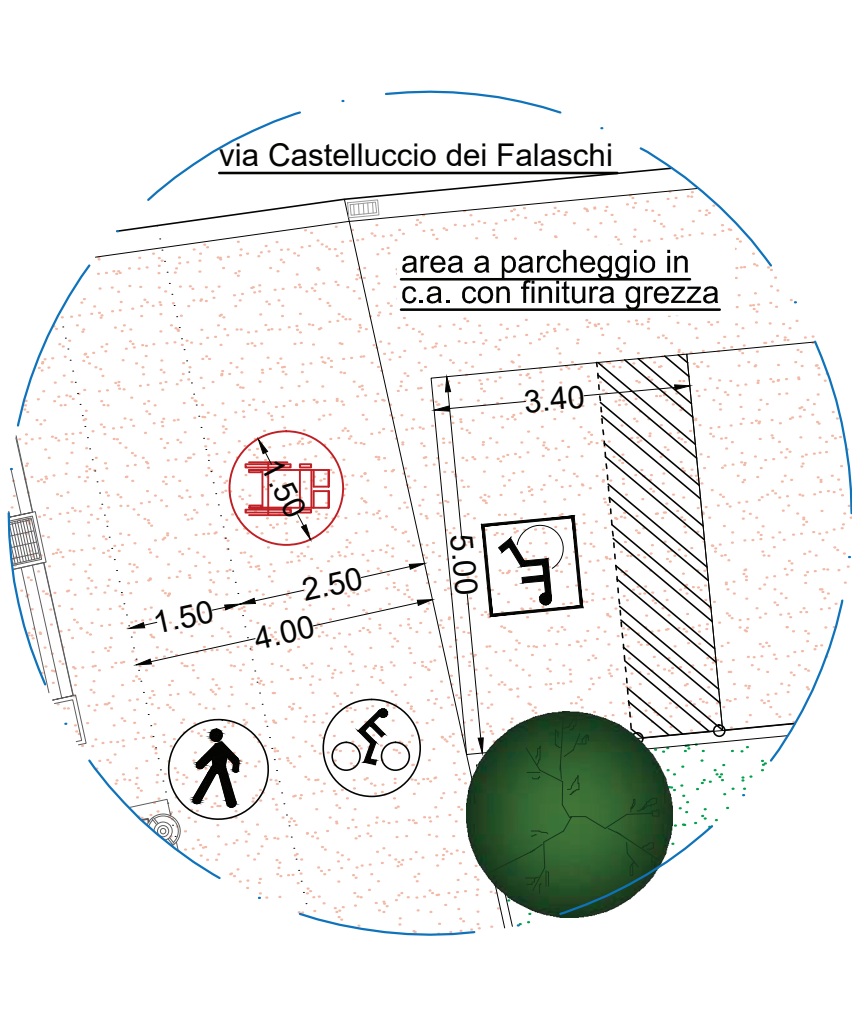
PART. 3- Parcheggio Scala 1:100
