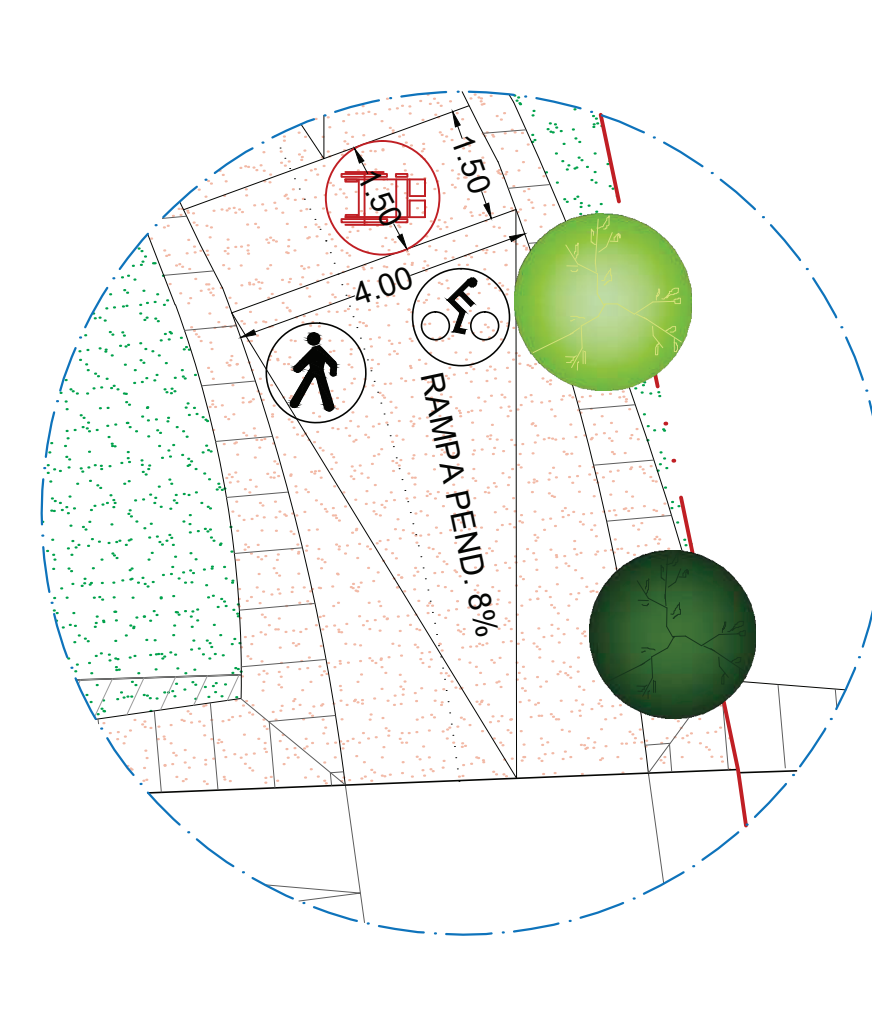
PART. 4- Rampa per accesso a verde primario Scala 1:100
