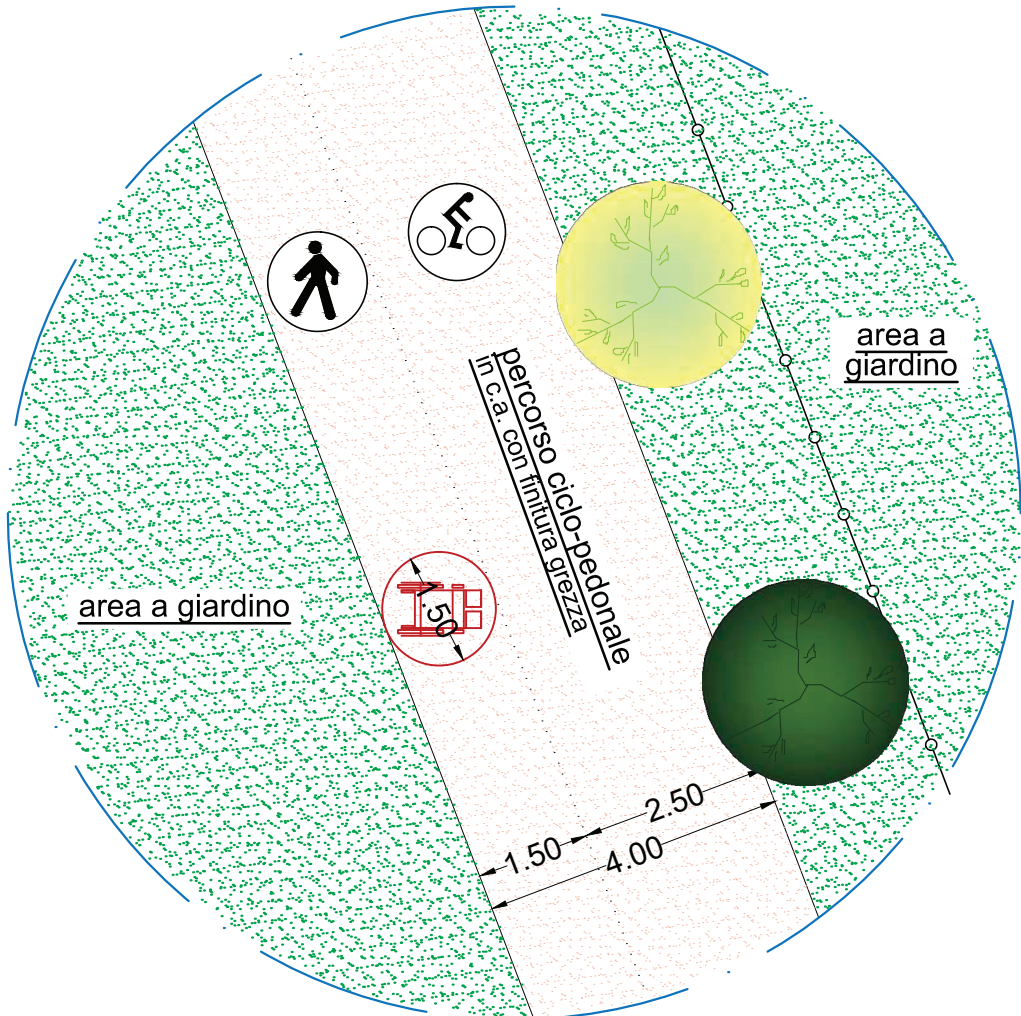
PART. 2- Percorso ciclo-pedonale Scala 1:100
