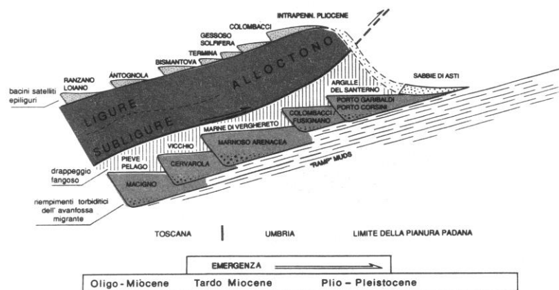
La figura illustra la progressione nell'avanzamento verso NE dell'alloctono Ligure e Subligure sulle successioni delle avansosse torbiditiche dei differenti domini. I sedimenti depositi direttamente sulla coltre ligure formano le successione dei bacini satellite epiligruri.
