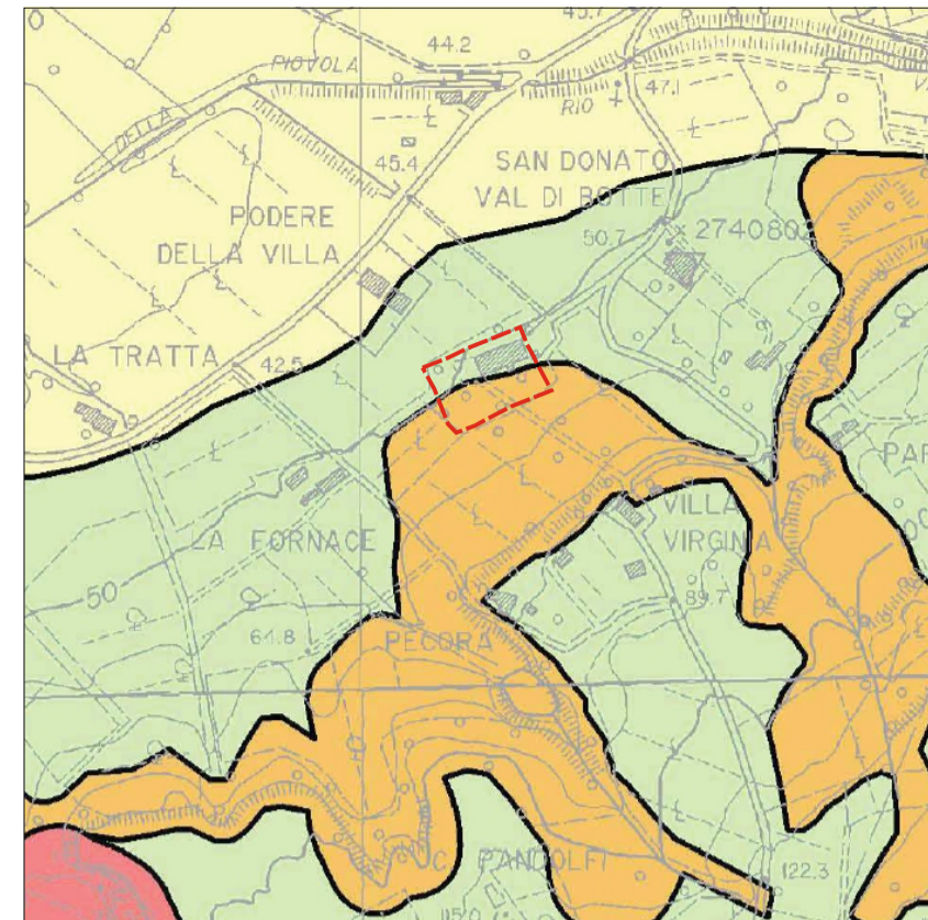
Carta della Pericolosità geomorfologica (Piano Strutturale)
