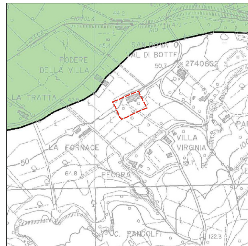
Carta della Pericolosità sismica (Piano Strutturale)
