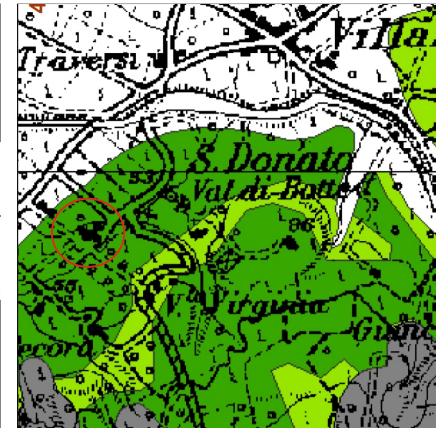
Perimetrazione delle aree con pericolosità da fenomeni geomorfologici di versante- Livello di Sintesi (Piano Stralcio Assetto Idrogeologico Autorità di Bacino del F. Arno)
